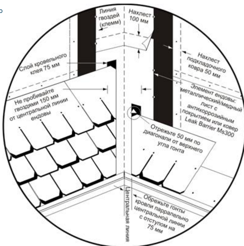
Рисунок 17-11. Устройство ендовы для Grand Manor
