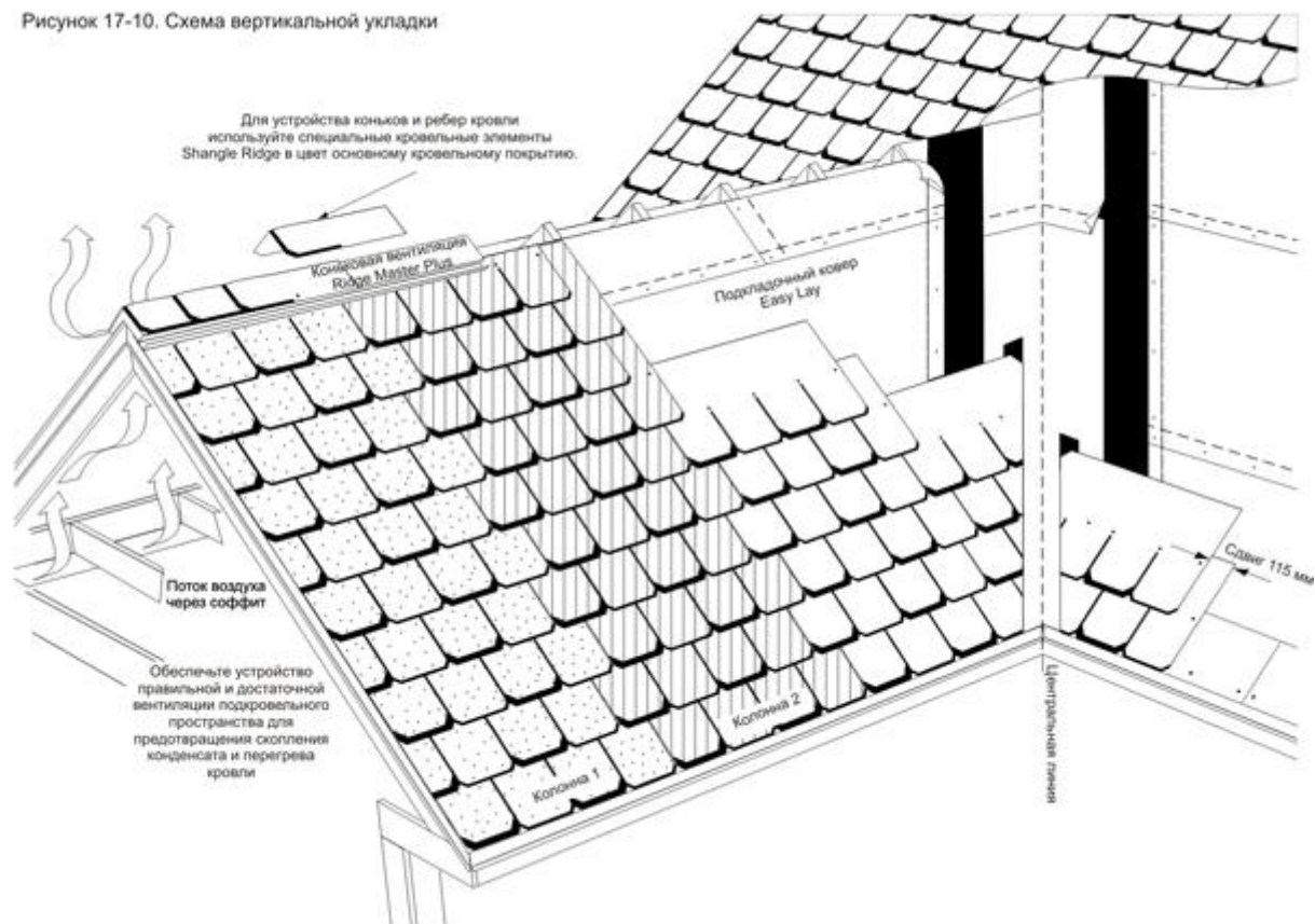
Рисунок 17-10. Схема вертикальной укладки
